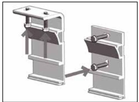
Abb. Decken- bzw. Wandkonsole
