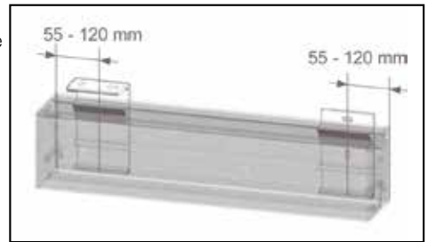
Abb. Decken- bzw. Wandkonsole
